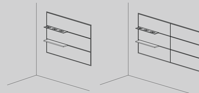
Telaio in alluminio H 135 sospeso per 3 elementi H 135 Aluminium frame suspended for 3 panels L. 150/200/300/400 - H. 135
